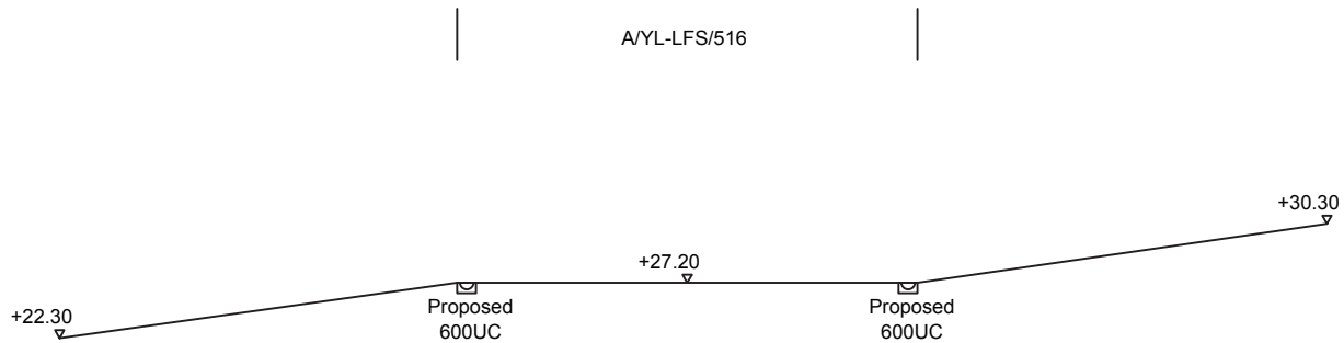
SECTION A-A
